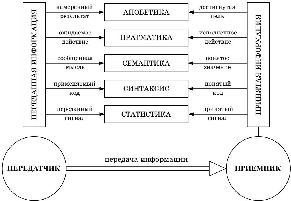
Рис. 4.3. Пять иерархических уровней информации
