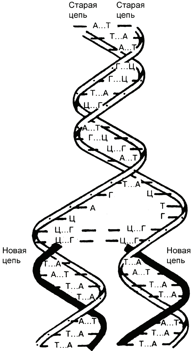
Рис. 4.2. Молекула ДНК и схема репликации ДНК
