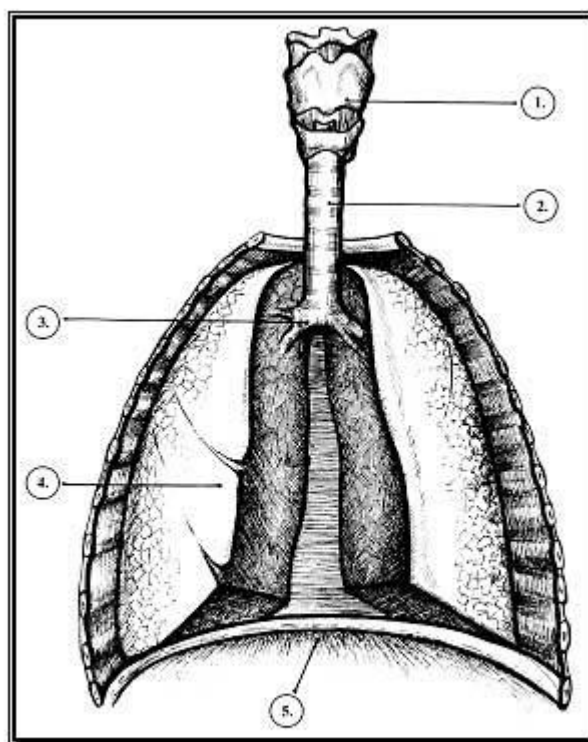
Рис. 1 Звукопроизводящий аппарат.
